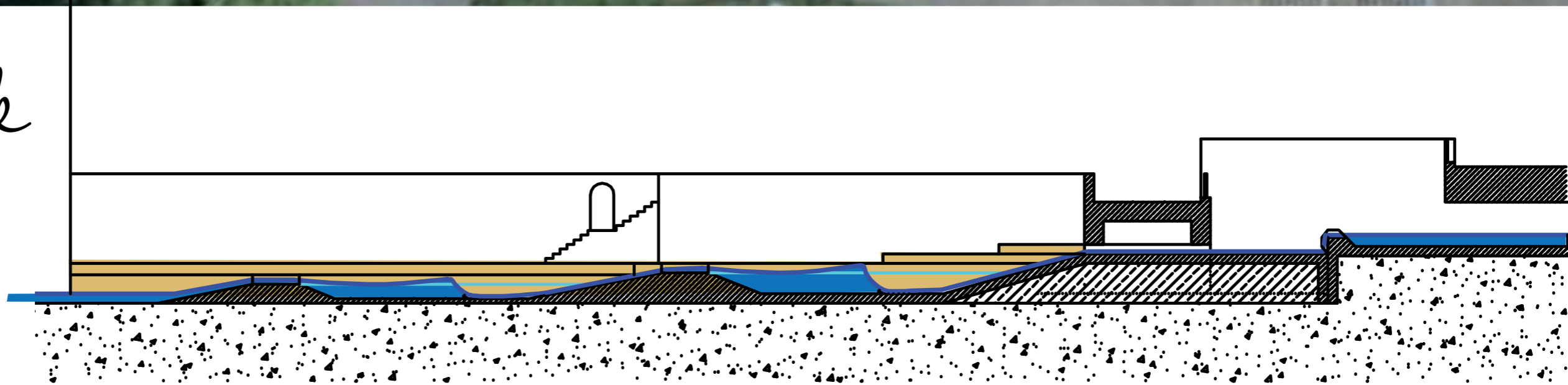
Prinzipskizze für eine artifizielle doppel Flusswelle zum Surfen in der Leine in Schnitt und Aufsicht M 1:200
